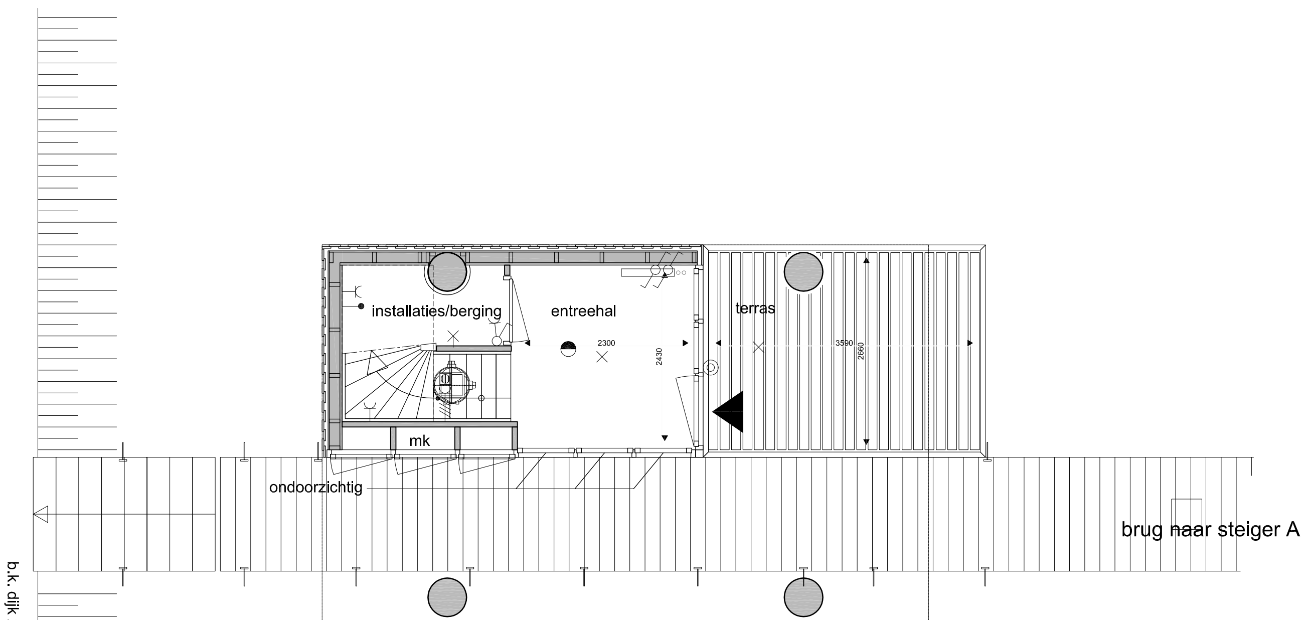
bouwnummer 13 plattegrond begane grond Lighthouse
